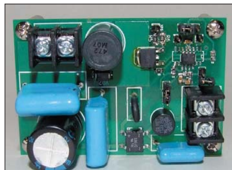
Рис. 1. Внешний вид платы для контроллеров AN9910 и AN9910B
