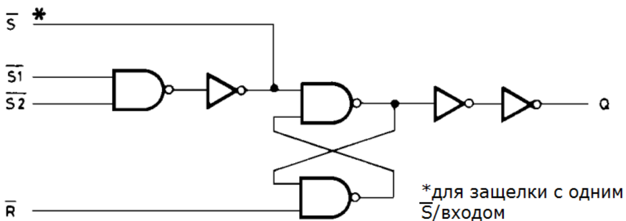
рисунок 1 – Схема функциональная
