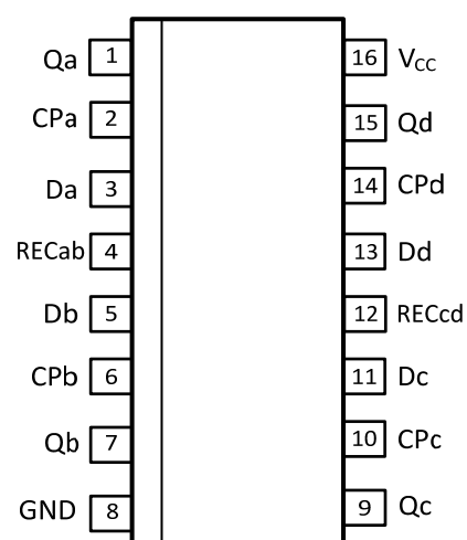
рисунок 4 конфигурация выводов SOP-16
