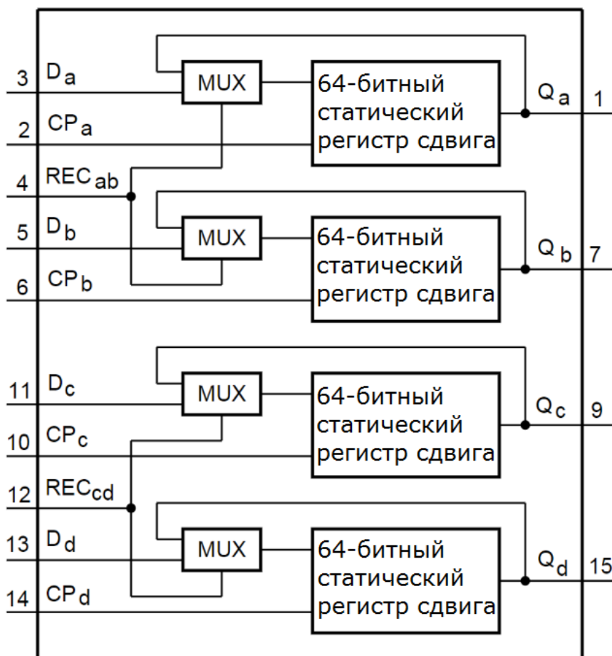
рисунок 1 – Схема функциональная
