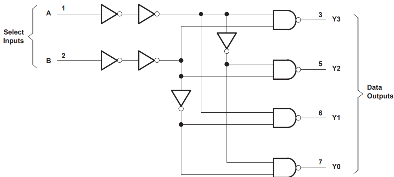
рисунок 1 – Схема функциональная
