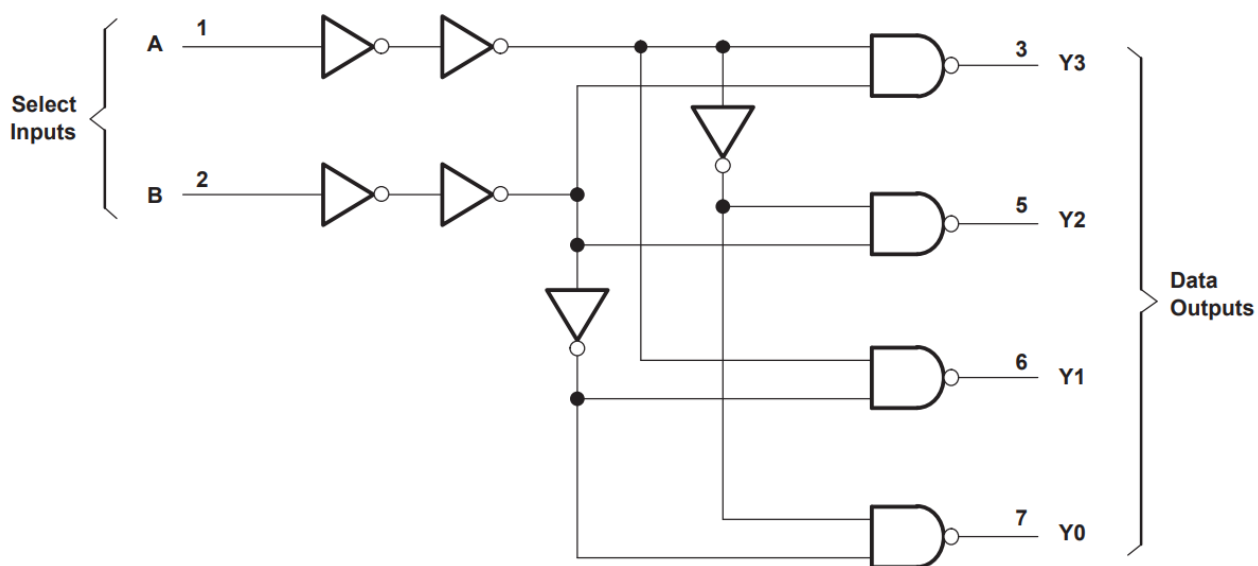
рисунок 1 – Схема функциональная
