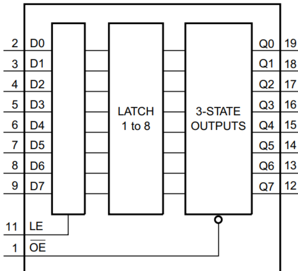
рисунок 1 – Схема функциональная
