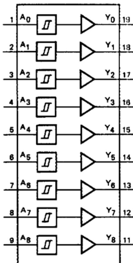
рисунок 1 – Схема функциональная
