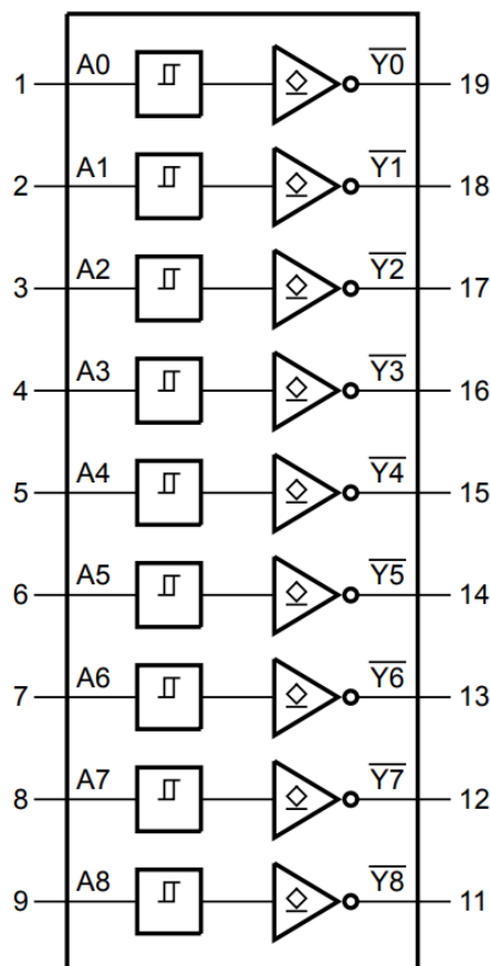
рисунок 1 – Схема функциональная
