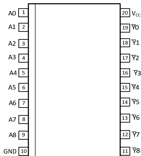
рисунок 5 конфигурация выводов SOP-20
