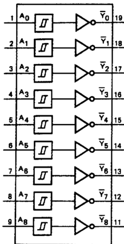
рисунок 1 – Схема функциональная
