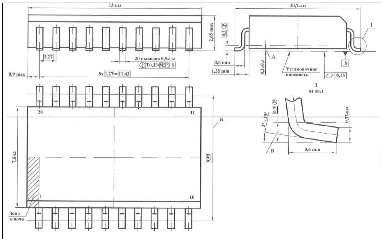
Корпус SOP-20(4321.20-А) (20 выводов), металлополимерный
