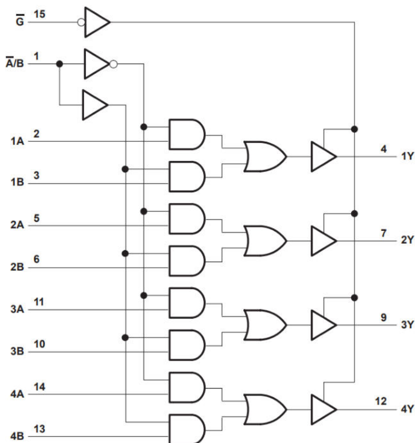
рисунок 1 – Схема функциональная
