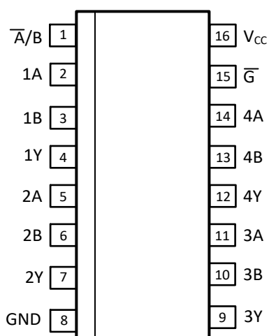
рисунок 2 конфигурация выводов SOP-16
