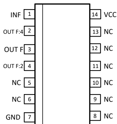
рисунок 2 конфигурация выводов SOP-14
