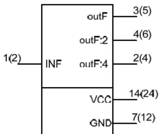
рисунок 1 – Схема функциональная
