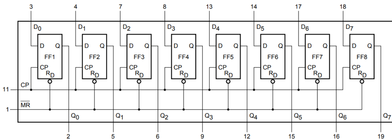
рисунок 1 – Схема функциональная
