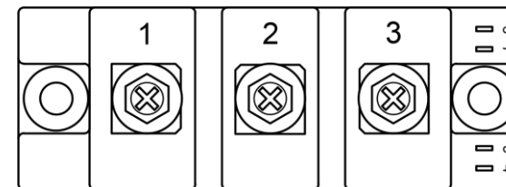
Рисунок 2 – Схема расположения выводов модулей AnDM100EA17M, AnDM100CA17M, AnDM100AA17M
