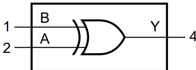
рисунок 1 – Схема функциональная
