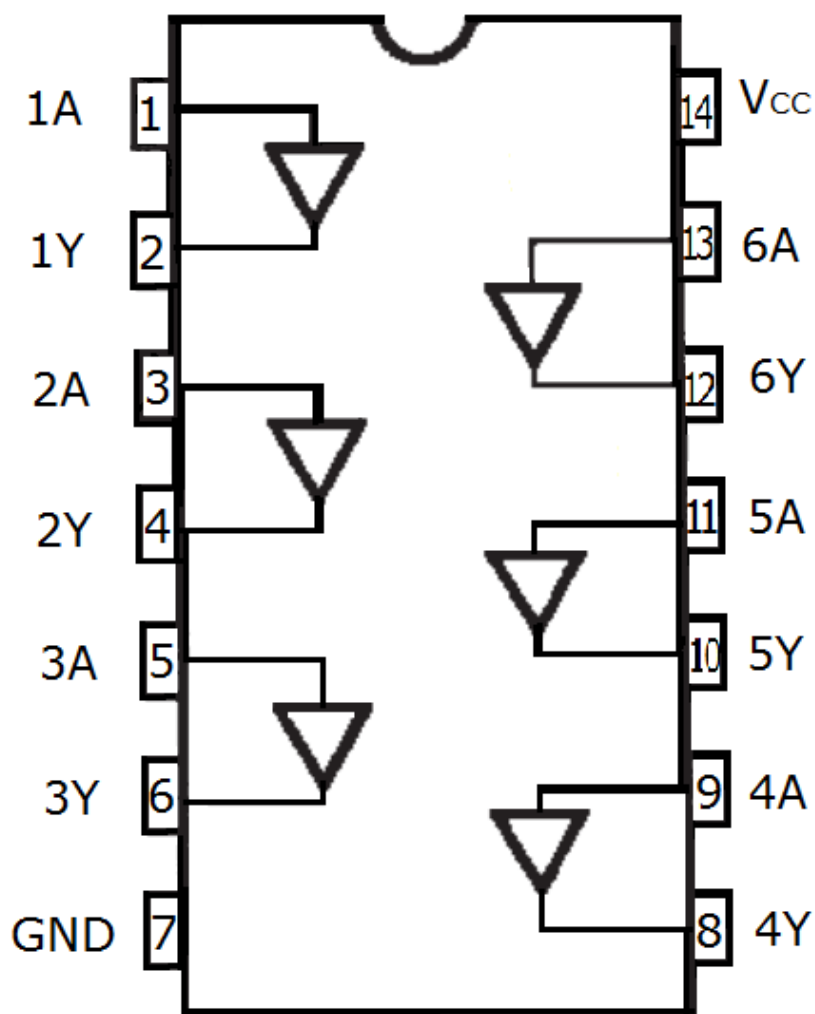
рисунок 1 – Схема функциональная
