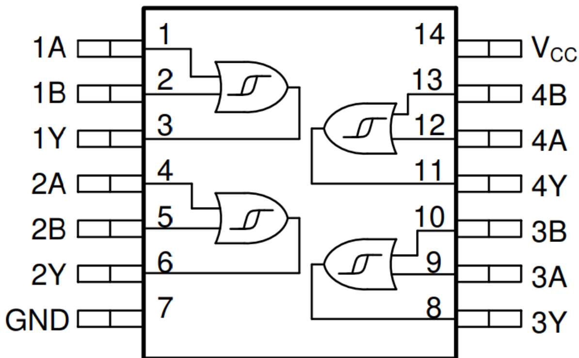
рисунок 1 – Схема функциональная
