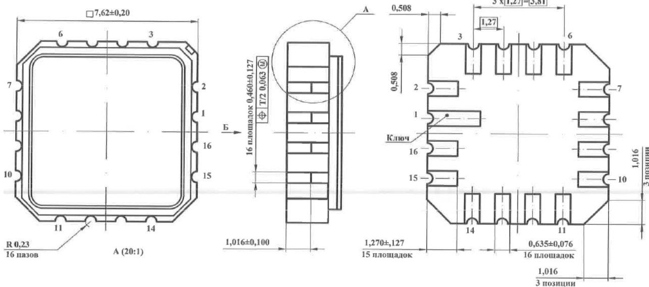
Корпус 5119.16-А (16 выводов), металлокерамический
