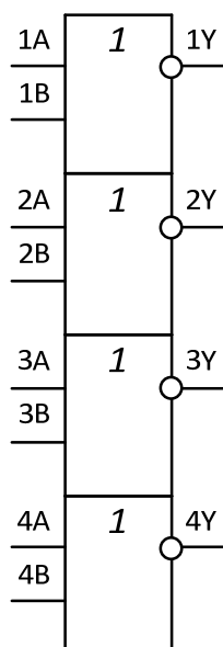
рисунок 1 – Схема функциональная
