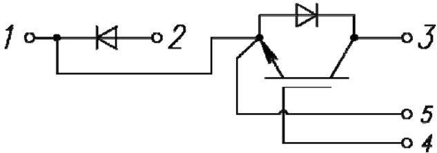
Рисунок 2 – Схема расположения выводов модулей AnM100RCA17M
