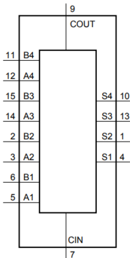
рисунок 1 – Схема функциональная
