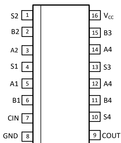
рисунок 2 конфигурация выводов SOP-16
