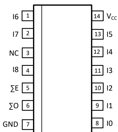
рисунок 2 конфигурация выводов SOP-14
