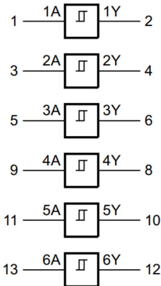
рисунок 1 – Схема функциональная
