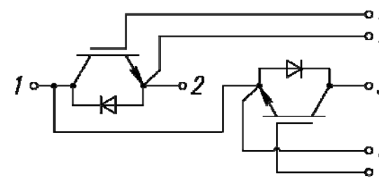
Рисунок 2 – Схема расположения выводов модулей AnM300HVB12M
