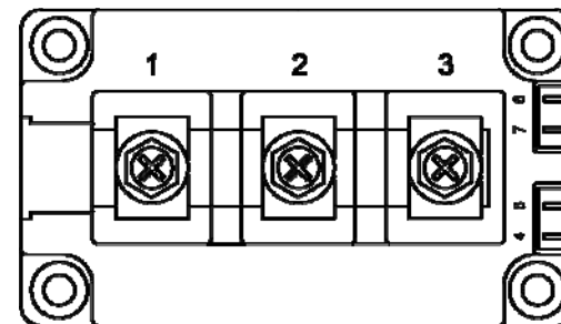
Рисунок 2 – Схема расположения выводов модулей AnM300HVB12M
