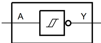
рисунок 1 – Схема функциональная
