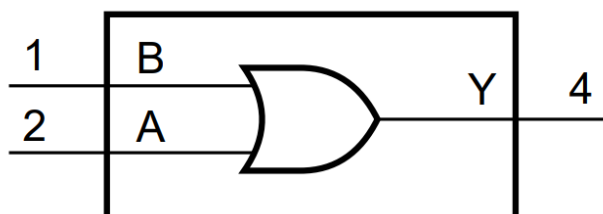
рисунок 1 – Схема функциональная
