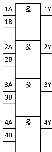
рисунок 1 – Схема функциональная
