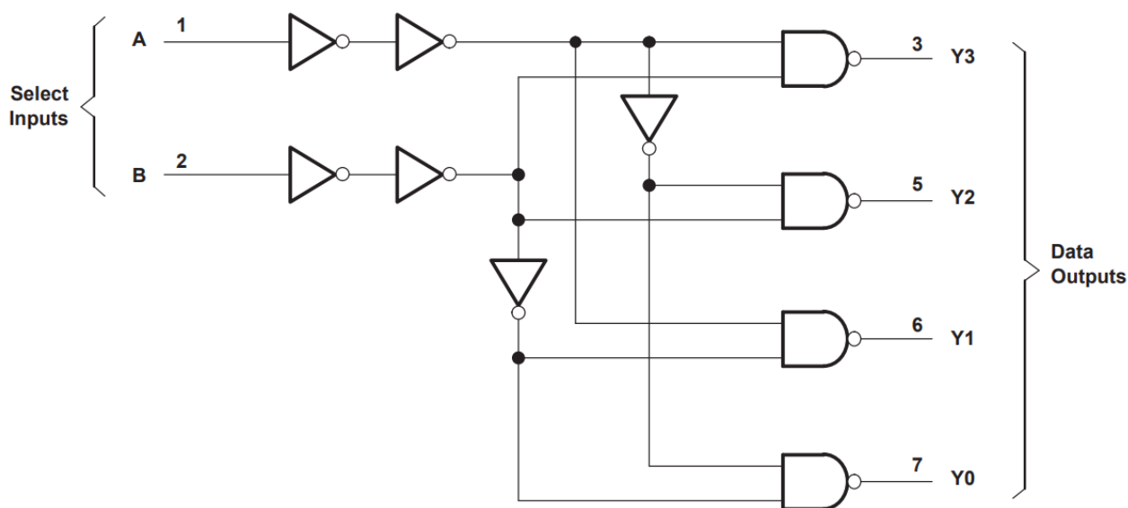
рисунок 1 – Схема функциональная
