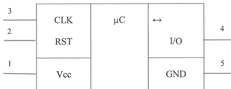
Рисунок 3 – Условное графическое обозначение для микросхем К5004ВЕ1АН4
