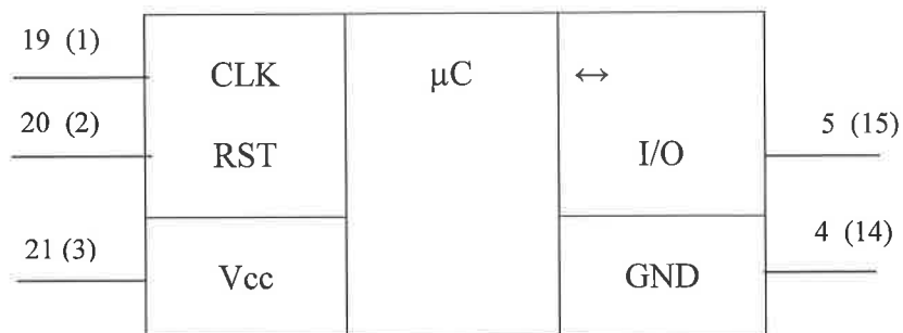
Рисунок 2 – Условное графическое обозначение для микросхем К5004ВЕ1АУ, К5004ВЕ1БУ, (К5004ВЕ1АУ1)
