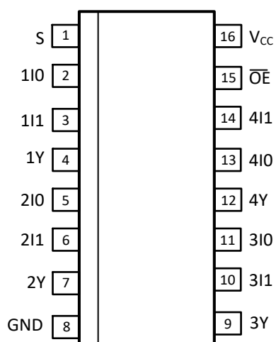
рисунок 2 конфигурация выводов SOP-16
