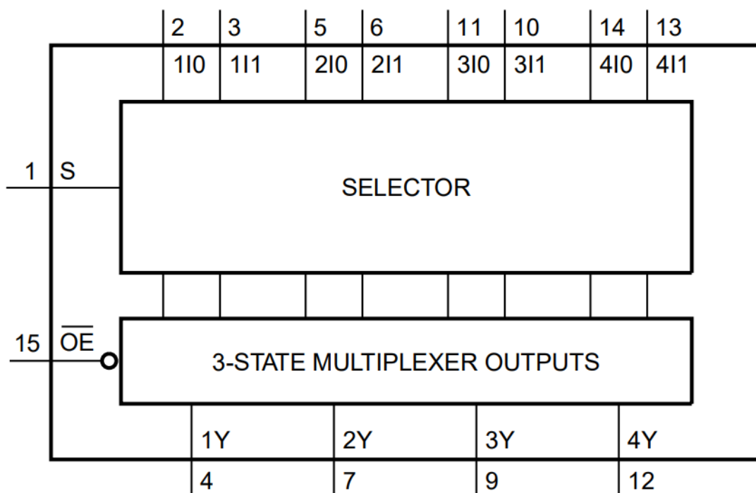
рисунок 1 – Схема функциональная
