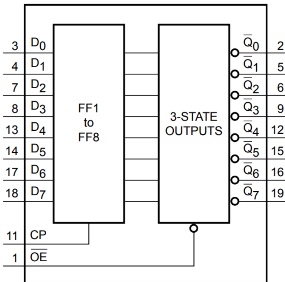
рисунок 1 – Схема функциональная
