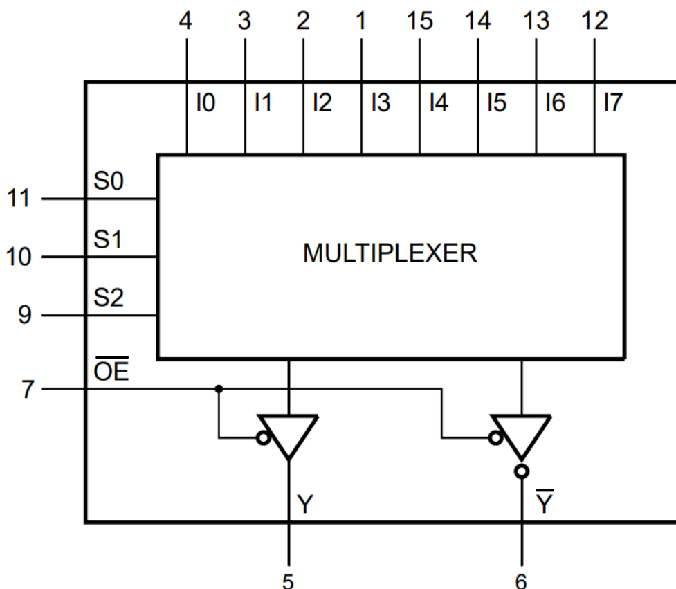
рисунок 1 – Схема функциональная
