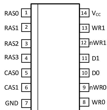
рисунок 4 конфигурация выводов SOP-14
