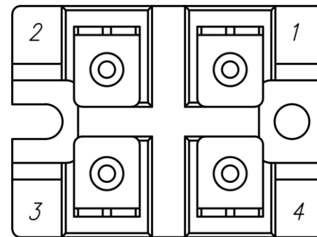
Обозначение выводов показано условно Рисунок 2 – Общий вид диодов AnSA50FRD12, AnSF50FRD12 с указанием расположения выводов
