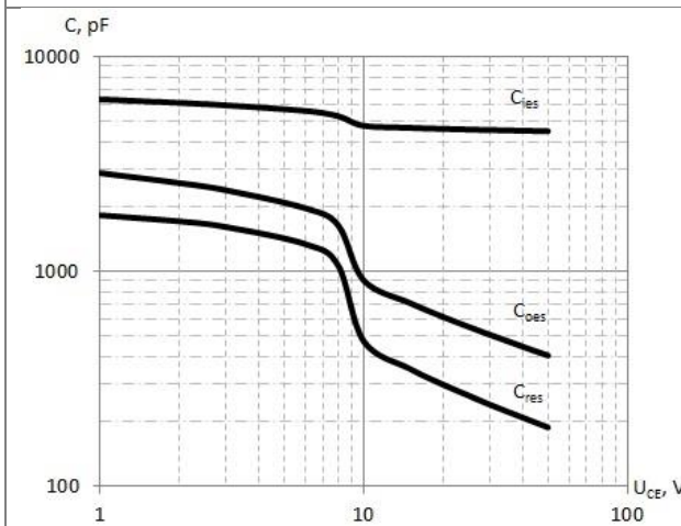
Рис.3 – Типовые зависимости входной C_{ies} , выходной C_{oes} , проходной C_{res} емкостей от напряжения коллектор эмиттер U_{CE}
