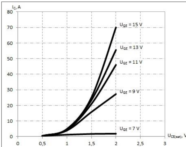
Рис.1 – Типовая выходная характеристика, T_J = 25\text{ }^{\circ}\text{C}
