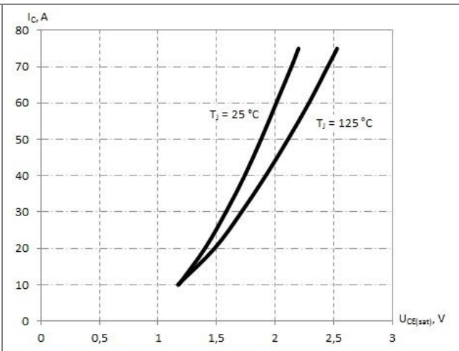
Рис.2 – Типовая характеристика напряжения насыщения от тока коллектора, T_J = 25 и 125\text{ }^{\circ}\text{C}
