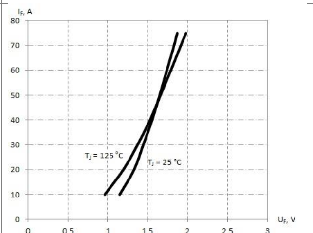
Рис.4 – Типовая зависимость прямого напряжения от прямого тока, T_J = 25 и 125\text{ }^{\circ}\text{C}
