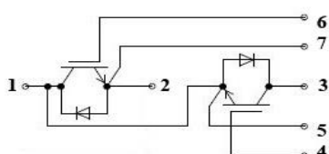
Полумост Half-Bridge
