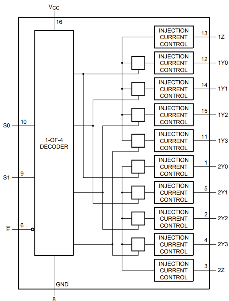
рисунок 1 – Схема функциональная
