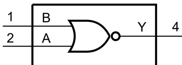
рисунок 1 – Схема функциональная
